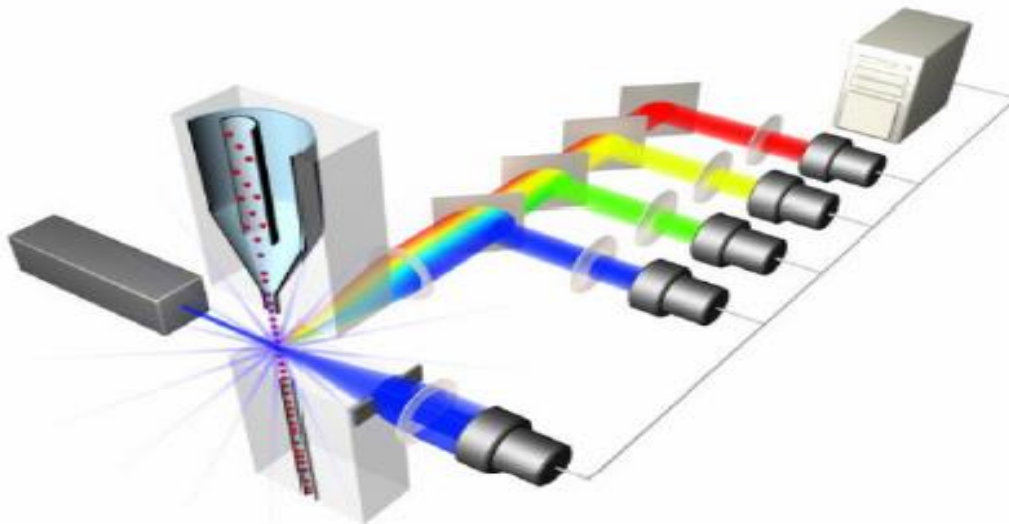
Figura 3. Luz do laser incidindo sobre a partícula da amostra de leite corada e detecção da luminescência
